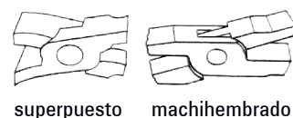
superpuesto machihembrado
